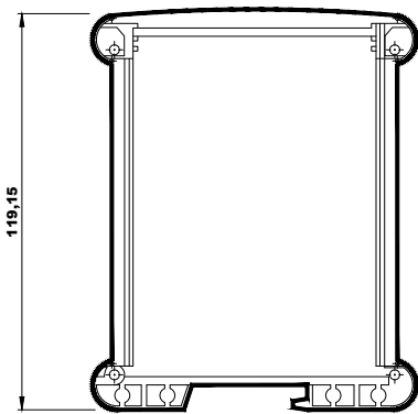
SECCIÓN A-A
