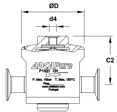
Optional dome-loading
